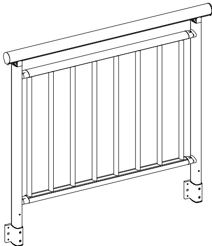
Tipo de fijación frente losa
