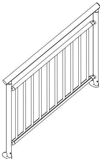
Tipo de fijación encima de losa
