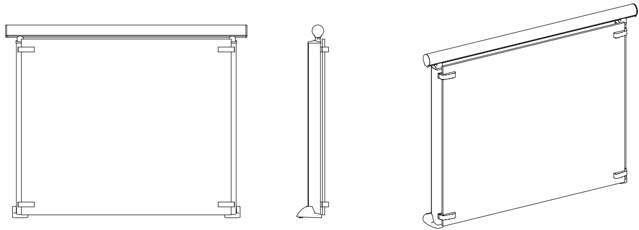
Tipo de fijación encima de losa
