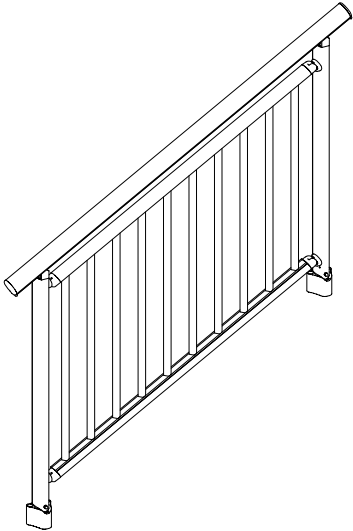
Tipo de fijación encima de losa
